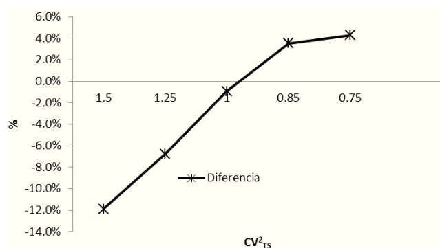
Figura 3. Diferencia vs CV_{T_s}^2
