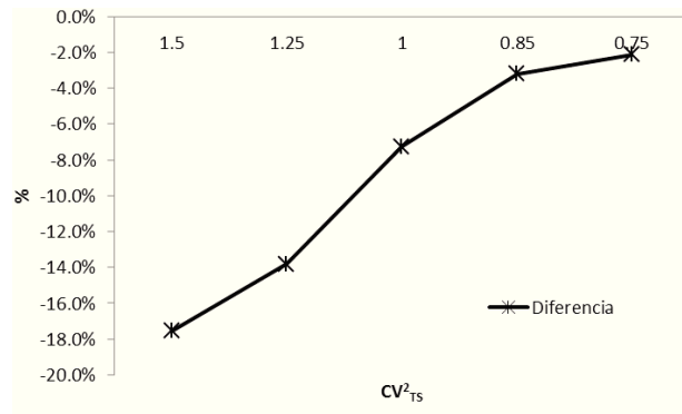
Figura 5. Diferencia vs CV_{T_s}^2 con cuello de botella
